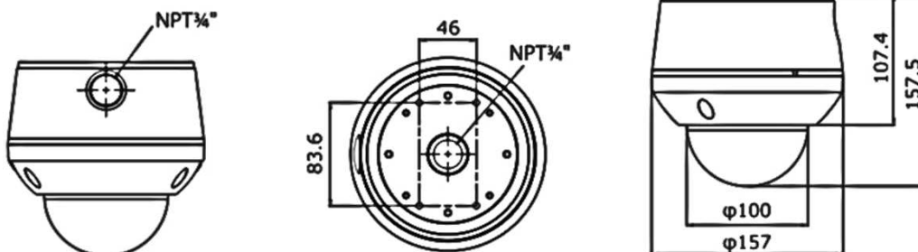
<外形寸法図> (mm)
